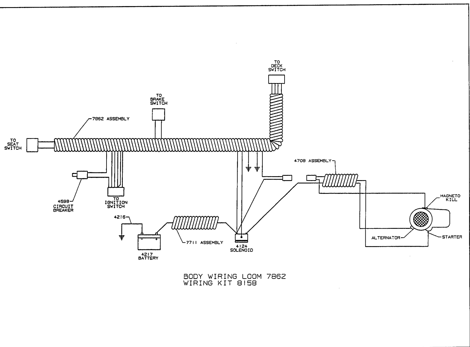
1995 Wiring Assembly Model ZTR 3303 / ZTR 3304
