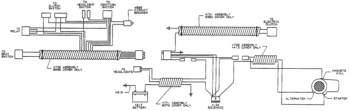
BODY WIRING LOOM - 4730
