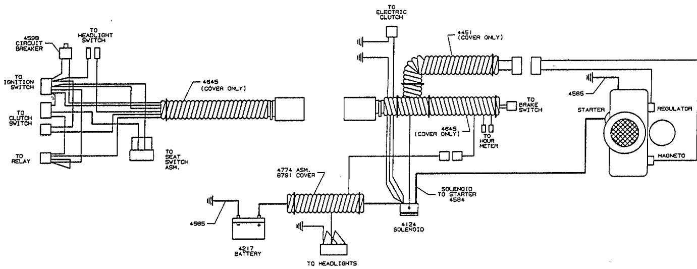
UPPER WIRING LOOM - 4728
