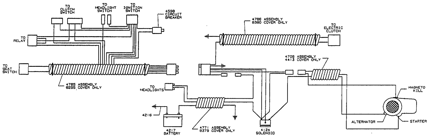
BODY WIRING LOOM - 4785
